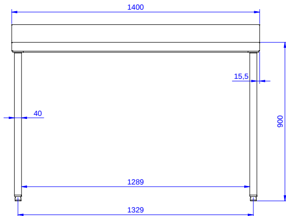
Alzado
